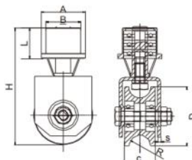
带导向弹簧滑轮 碳钢 & 304
