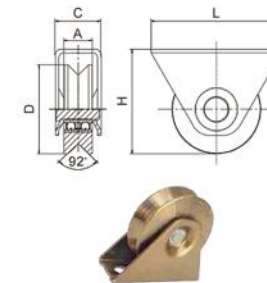
梯形V槽双轴承滑轮
