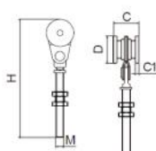
圆板两轮挂轮 (小) Hanging Door Roller (2 Rollers)
