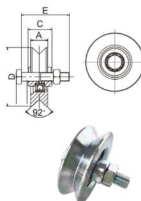
带螺杆V槽单轴承滑轮
