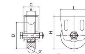
U槽可调滑轮
