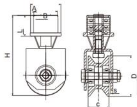
带导向弹簧滑轮 碳钢 & 304
