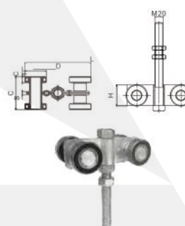
合板轴承挂轮 Hanging Door Roller (4 Rollers)
