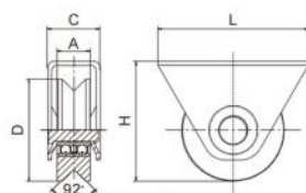
V槽半圆双轴承滑轮 (南美)
