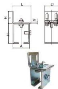
尖槽挂轮轨道 Hanging Door Roller Rail
