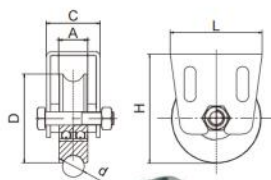
U槽可调滑轮
