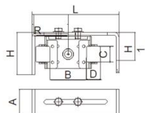
双轮可调上门兜 Guide bracket
