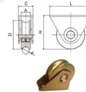
梯形U槽双轴承滑轮
