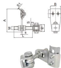
M16长杆双调节铰链 Adjustable Gate Hinge
