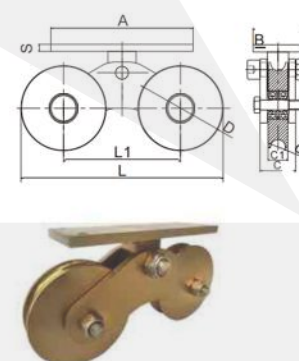
重型双轮滑轮
