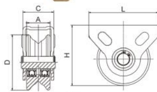
特殊滑轮
