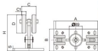
中五轮 5 Medium Wheels
