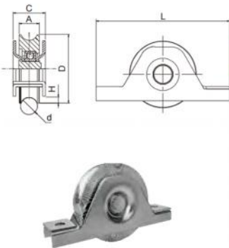
叠片U槽单轴承滑轮
