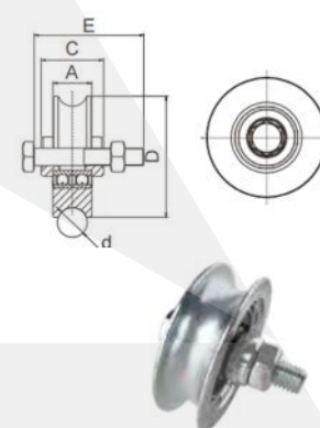
带螺杆U槽双轴承滑轮
