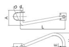
香蕉挂轮支架 Banana Hanger Bracket
