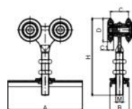
四轮轴承挂轮 Hanging Door Roller (4 Rollers, Forge Centre Plate)
