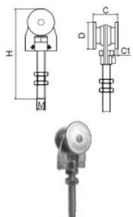
圆板两轮挂轮 (大) Hanging Door Roller (2 Rollers)
