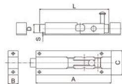
普通插销 Gate Latch
