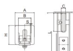
70x70五轮导轮 Guide Wheel
