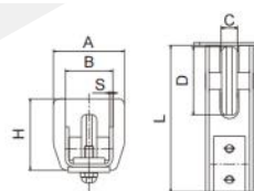
大五轮导轮 Guide Wheel
