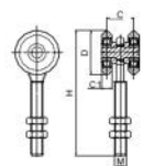
两轮轴承挂轮 Hanging Door Roller (2 Rollers, Forge Centre Plate)
