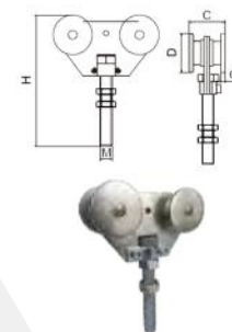
圆板四轮挂轮 (大) Hanging Door Roller (4 Rollers)
