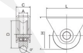
U槽半圆双轴承滑轮 (南美)
