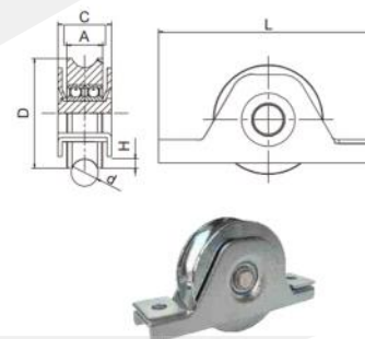
叠片U槽双轴承滑轮
