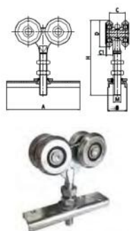
四轮轴承挂轮 Hanging Door Roller (4 Rollers, Forge Centre Plate)
