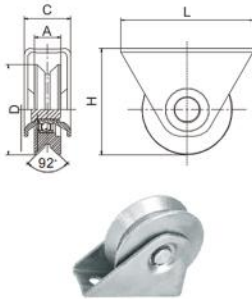
梯形Y槽单轴承滑轮
