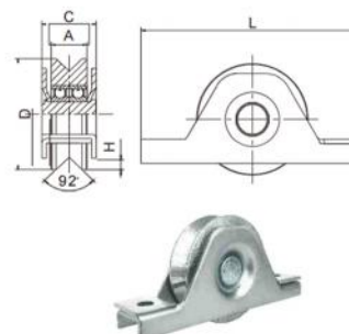
叠片V槽双轴承滑轮
