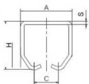
尖槽挂轮轨道 Hanging Door Roller Rail
