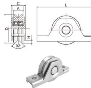
叠片Y槽双轴承滑轮
