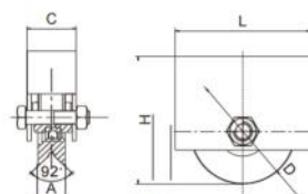
方形盒子单轴承Y槽滑轮
