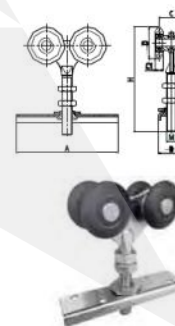
四轮尼龙挂轮 Hanging Door Nylon Roller (4 Rollers)
