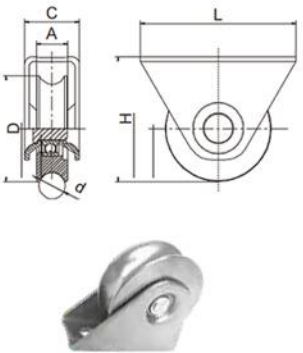
梯形U槽单轴承滑轮
