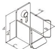
小五轮门兜 Gate Catcher
