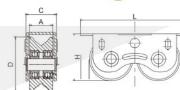
双轮特殊滑轮
