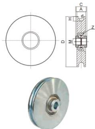
单槽单轴承滑轮
