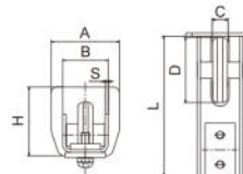
小五轮导轮 Guide Wheel
