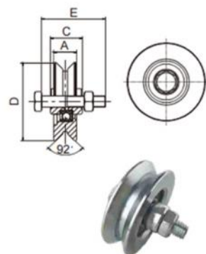
带螺杆Y槽单轴承滑轮
