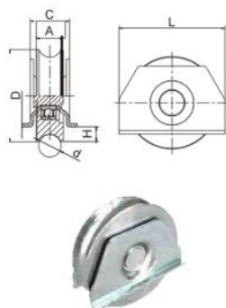
双片U槽单轴承滑轮
