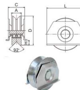
双片Y槽双轴承滑轮
