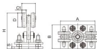
升降五轮 5 Wheels Simple
