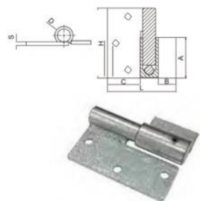
不对称蝶形铰链 Butt Hinge
