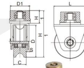
带导向轮滑轮
