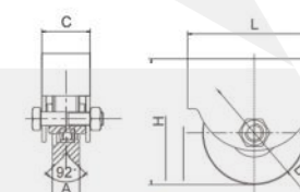
盒子单轴承Y槽滑轮
