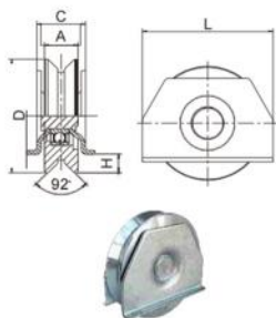
双片Y槽单轴承滑轮
