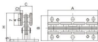
中八轮 8 Medium Wheels
