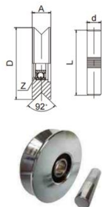
带轴单轴承滑轮
