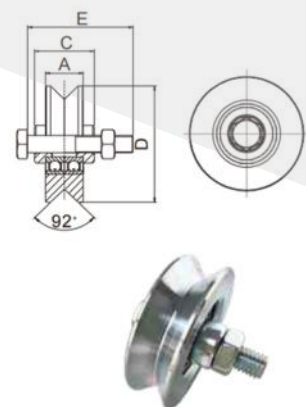
带螺杆V槽双轴承滑轮
