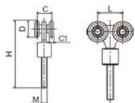
螺杆四轮挂轮 Hanging Door Roller (4 Rollers, with Bolt)
