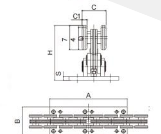
中十六轮 16 Medium Wheels
