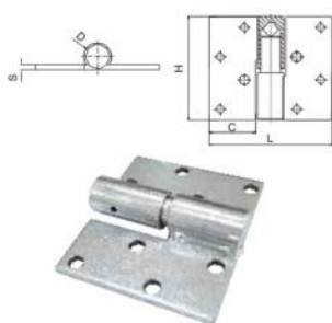
蝶形铰链 Butt Hinge
