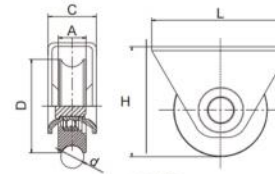
U槽半圆单轴承滑轮 (南美)
