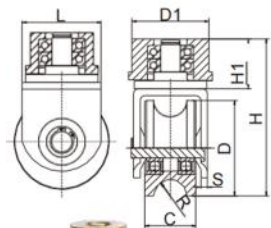
带导向轮滑轮
