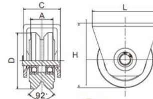
非洲双轴承滑轮
