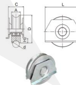
双片U槽双轴承滑轮
