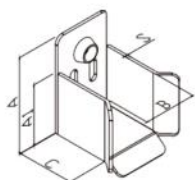
中八轮门兜 Gate Catcher
