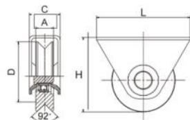
V槽半圆单轴承滑轮 (南美)
