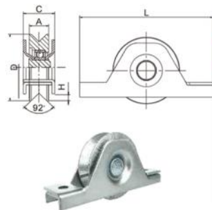
叠片V槽单轴承滑轮
