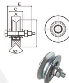
带螺杆Y槽双轴承滑轮
