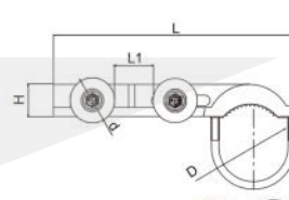
导轮
