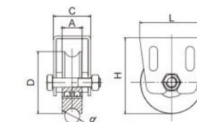
U槽可调滑轮
