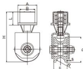
带导向弹簧滑轮 碳钢 & 304
