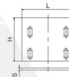
名称 -ARTICLE 4 Hole Purlin Clip
