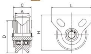
特殊滑轮
