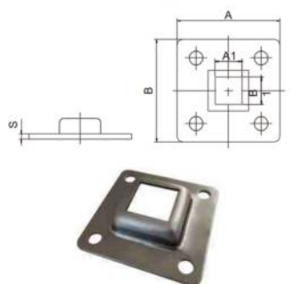
中间突出立柱底板 Steel Raised Base Plate
