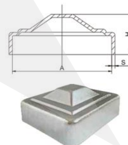
美国梯形柱盖 Square Steel Post Cap
