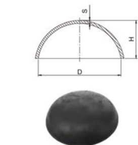
美国圆盘柱盖 Steel Post Cap
