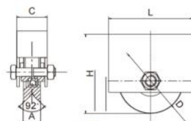
方形盒子单轴承Y槽滑轮
