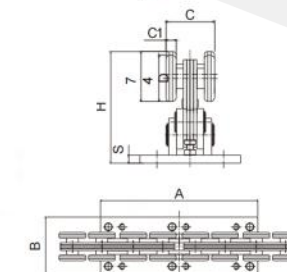
中十六轮 16 Medium Wheels
