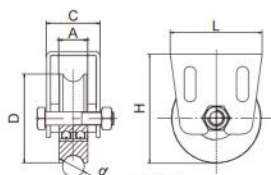
U槽可调滑轮
