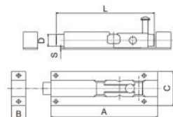
普通插销 Gate Latch
